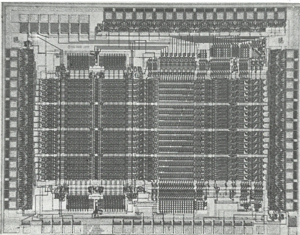
Un circuito sperimentale progettato al California Institute of Technology.
