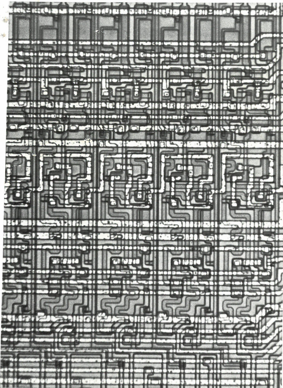
L'addizionatore elettronico della microfotografia qui sotto è una piccola porzione di un microelaboratore, realizzato sulla superficie di un chip di silicio.
